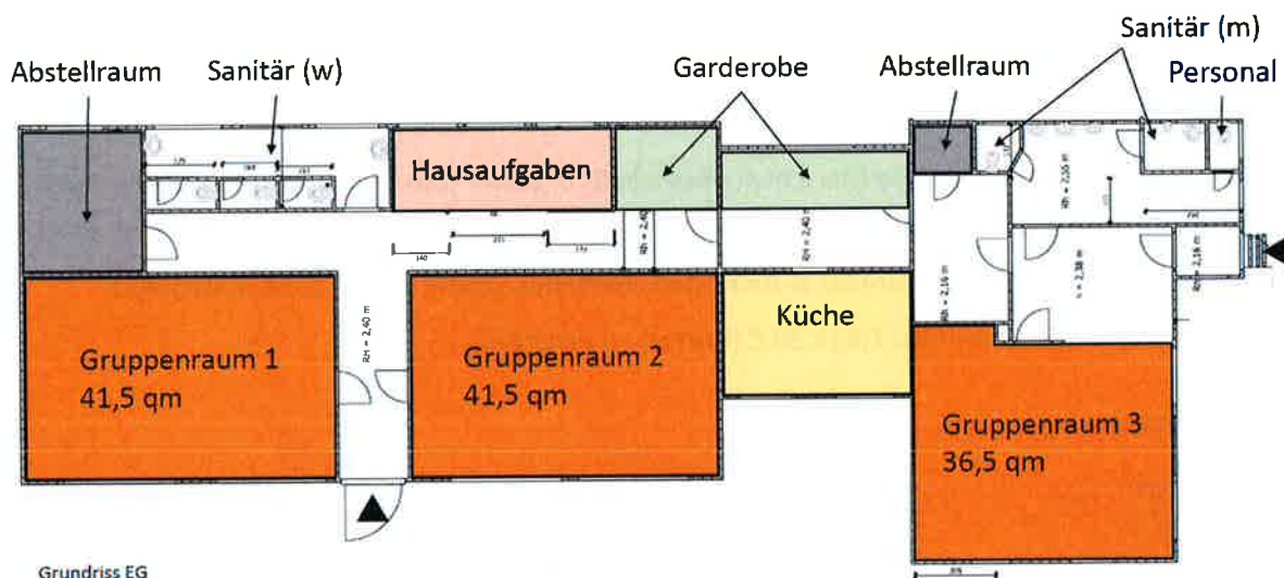
Grundriss EG ohne Maßstab Stand: 4.5.2022 Gemeinde Malschwitz Weißflog
